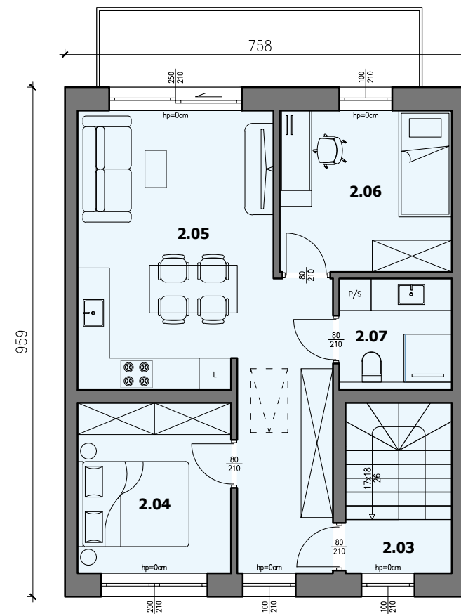
RZUT PIĘTRA
