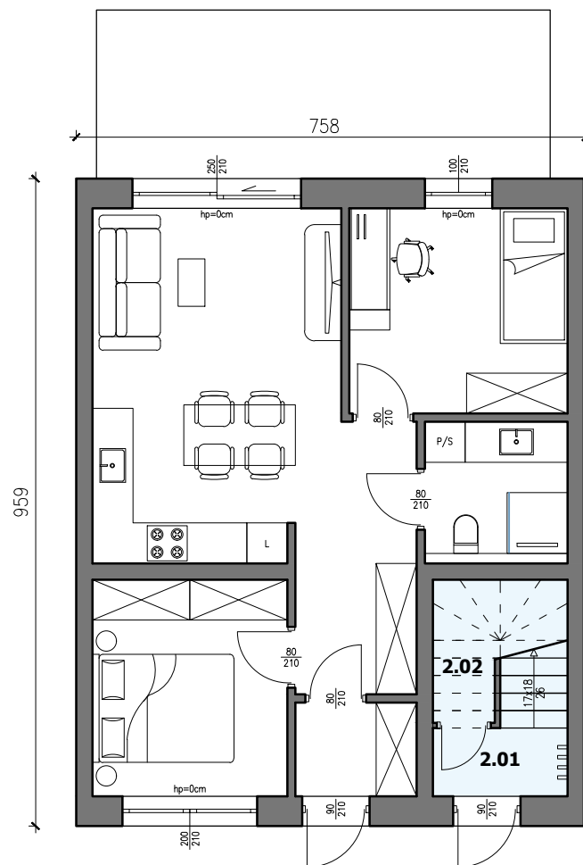
RZUT PARTERU
