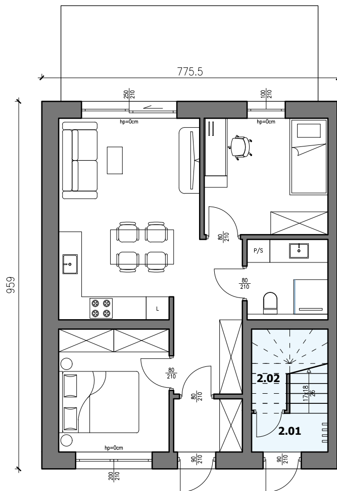
RZUT PARTERU
