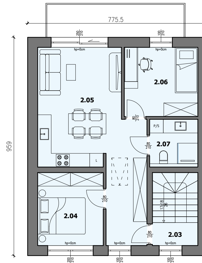
RZUT PIĘTRA
